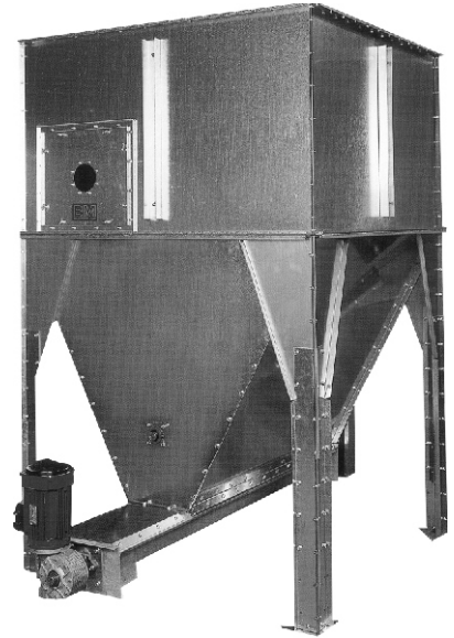
Rührwerk mit Schneckengetriebemotor 0,55 kW
