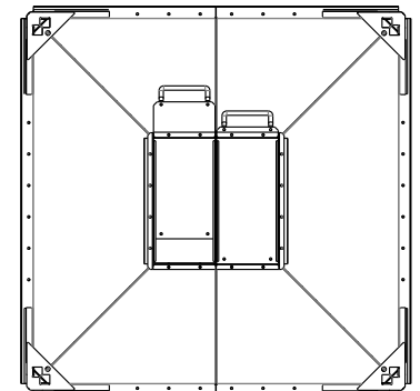
Abb: Silo Draufsicht, geteilter Schieber 500x500 mm
