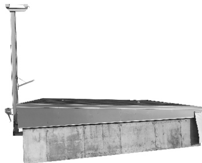
Abb: Gossendeckel 4,60x4,60m-nicht überfahrbar- mit Handwinde zum Öffnen
