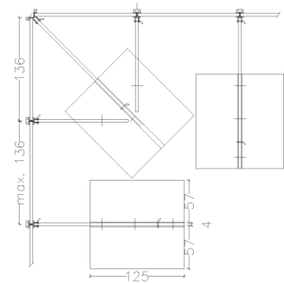
L-Stütze 4,0 m - Details / Beispiel
